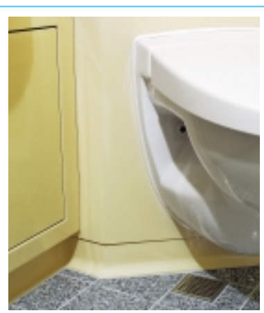
Risteilijän sviitin kylpyhuoneen lattia on graniittia. Graniitti on liimattu lujitemuoviseen lattiaelementtiin. Rakenne on vesitiivis ja hygieeninen.
